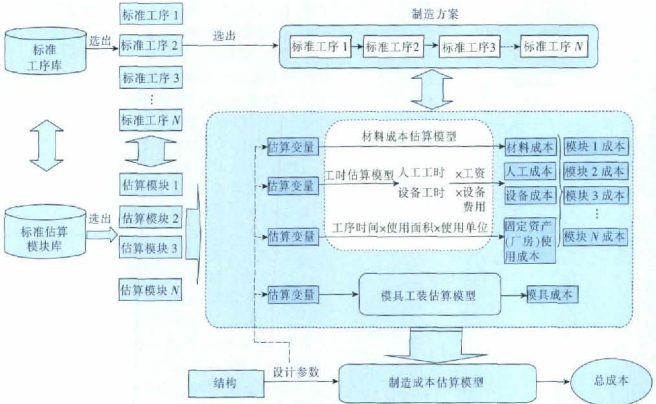
图2 复合材料结构制造成本估算框架
