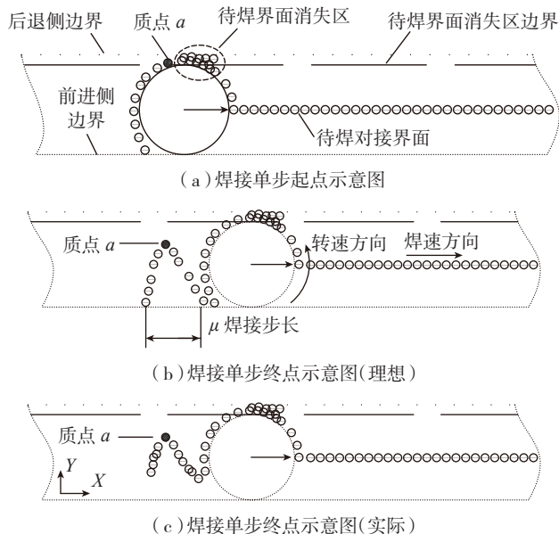
图2 XY平面S线特征模型
