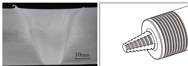
(a) 40mm 铝合金 FSW 焊核
