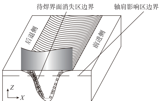
(a) 焊接单步起点示意图
