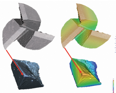
钻头的三维表面形貌测量
