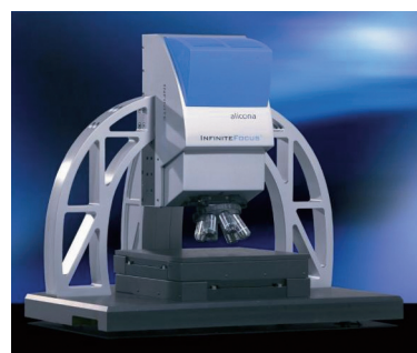
全自动变焦三维表面测量仪
