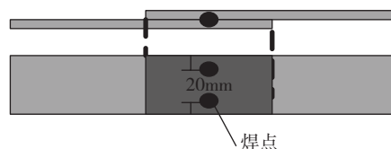
图2 点焊试验件
