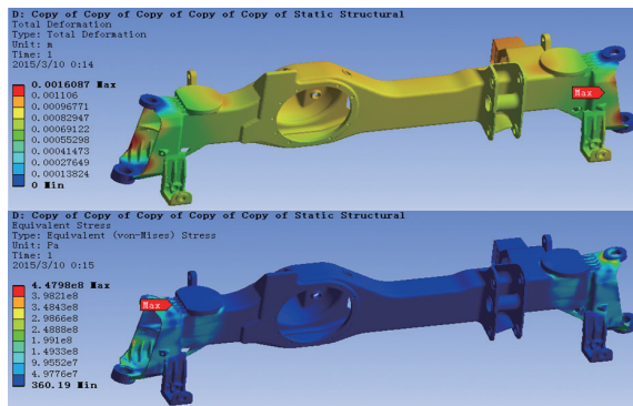
轻型前桥壳设计
